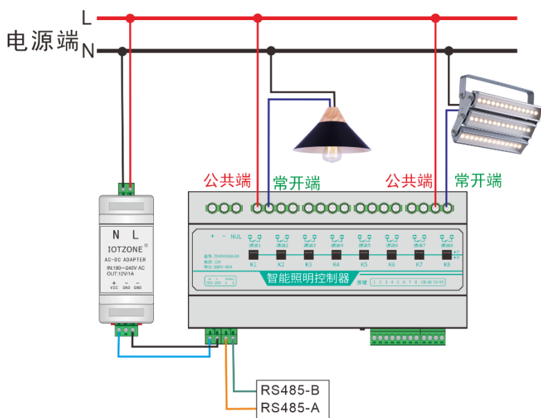
交流220V设备接线方法
