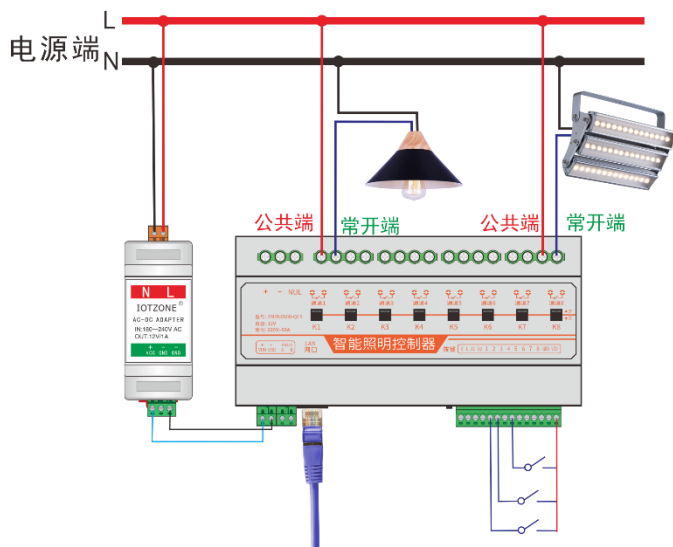
交流220V设备接线方法
